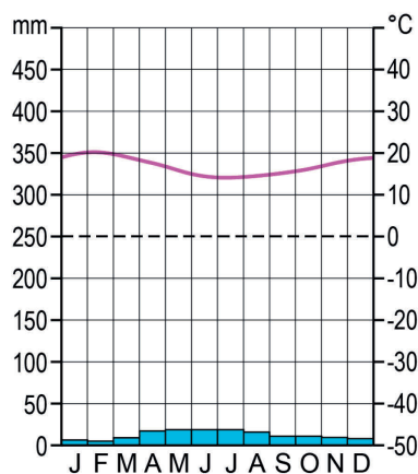
klimaatgrafiek a
