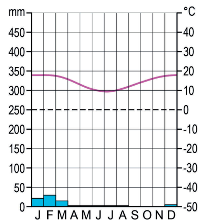
klimaatgrafiek c
