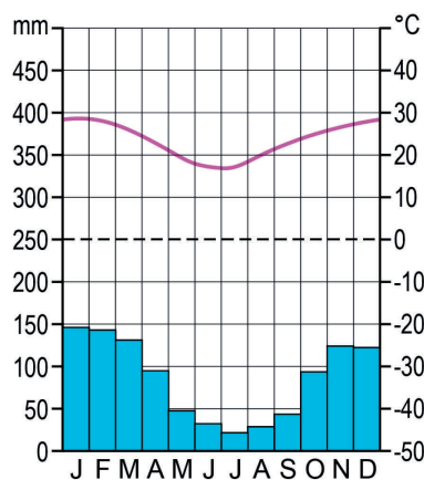
klimaatgrafiek b
